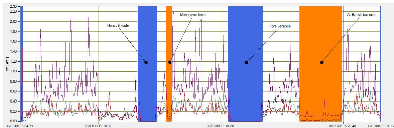
Niveaux d'accélération selon les 3 axes sur EvecViewerDuo ; les zones d'absence de l'opérateur apparaissent en bleu.
